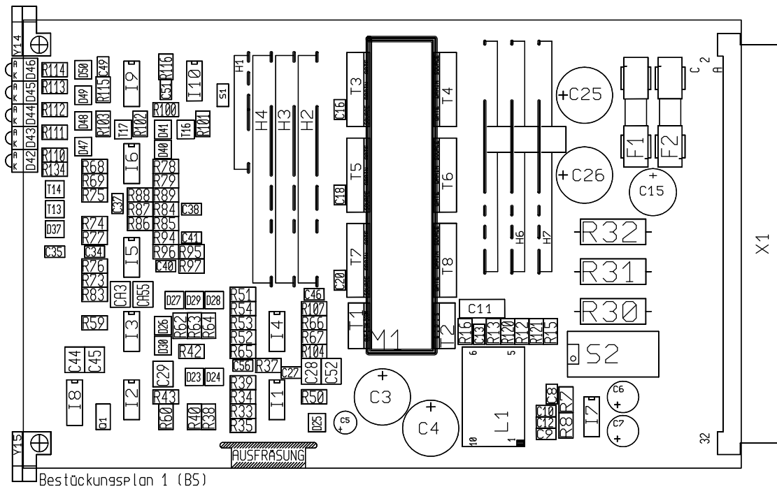
Bild 8 Lage der Sicherungen - Bestückungsplan MSK -
