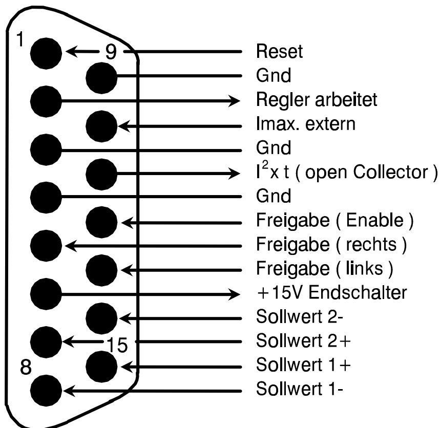
Lötseite des Gegensteckers
