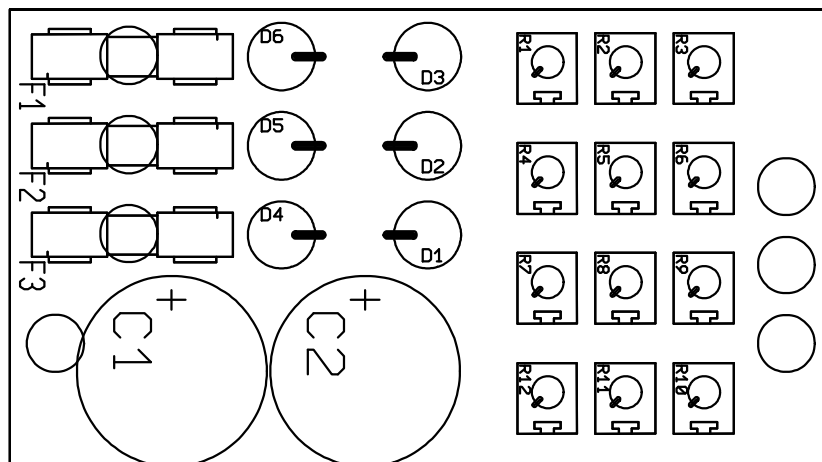
Bild 10 Bestückungsplan Option 24V ext + int. Bremswiderstände - Lage der Sicherungen -
