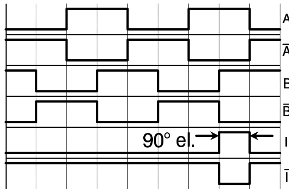
Bild 6 Impulsdiagramm bei Rechtslauf
