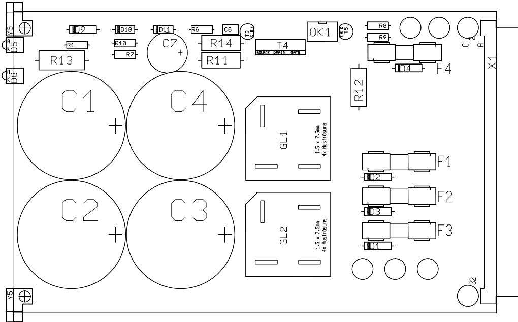
Bild 9 Lage der Sicherungen - Bestückungsplan MTB 25 -
