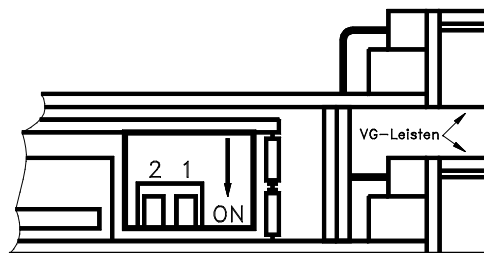
Bild 7 Lage der Schalter 1 und 2
