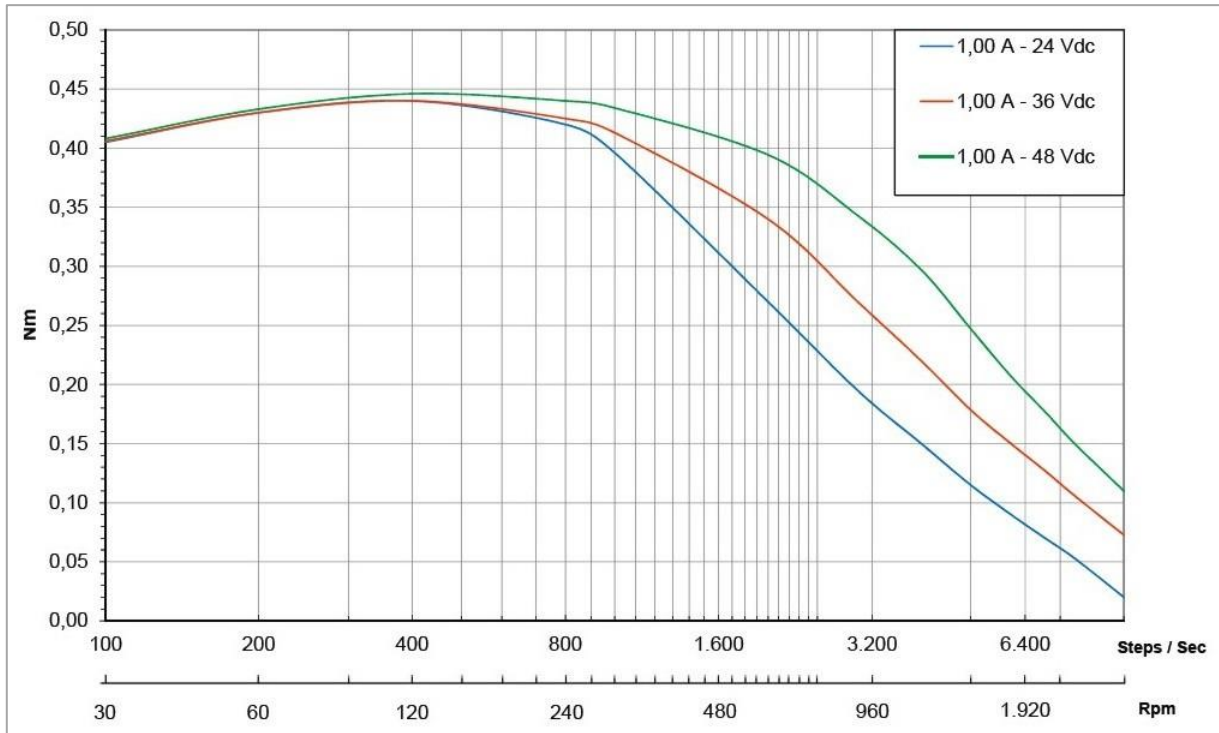
Drehmomentkennlinie HL13
