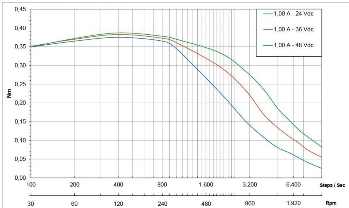
Drehmomentkennlinie HL12
