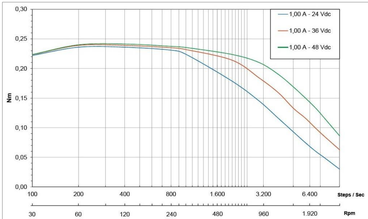
Drehmomentkennlinie HL11
