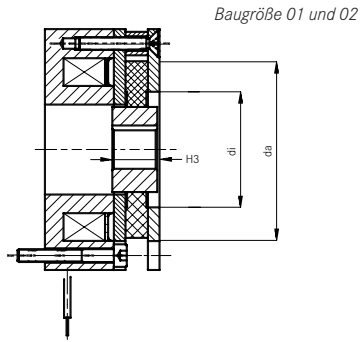
Anbau magnetgehäuseseitig
