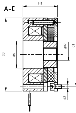
Anbau flanschseitig
