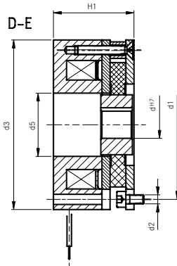
Anbau flanschseitig
