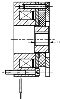
Baugröße 03 bis 05
